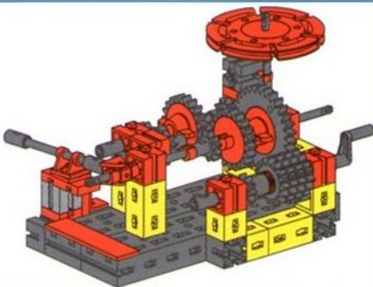
Schaltgetriebe / Transmission / Changement de vitesse / Schakelmechanisme / Cambio de marchas / Meccanismo di cambio 33
