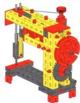
Nähmaschine / Sewing Machine / Ma- chine à coudre / Naaimachine / Ma- quina de coser / Maccina da cucire 81
